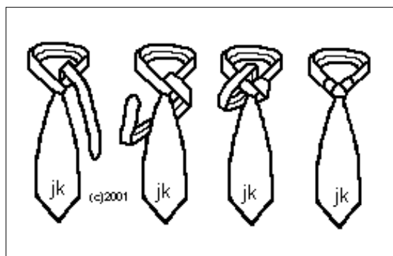
Atlantik Knoten
